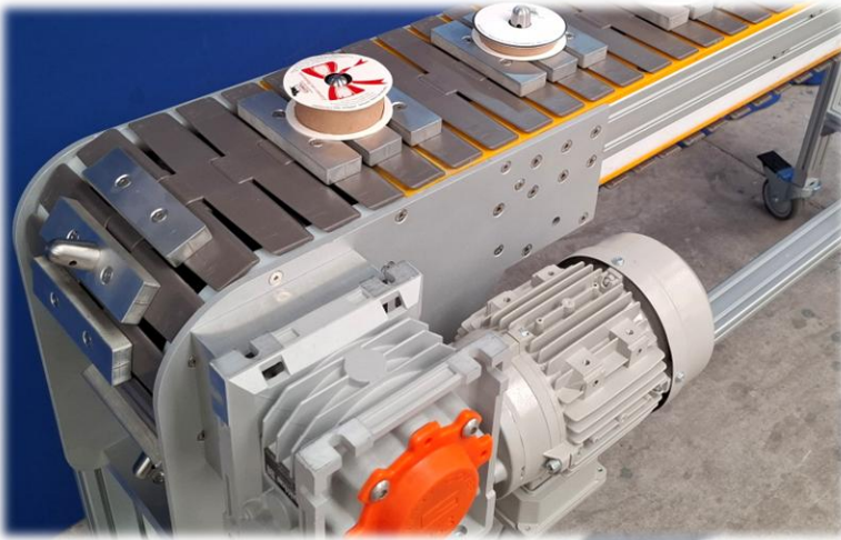
Cadena Plástica
